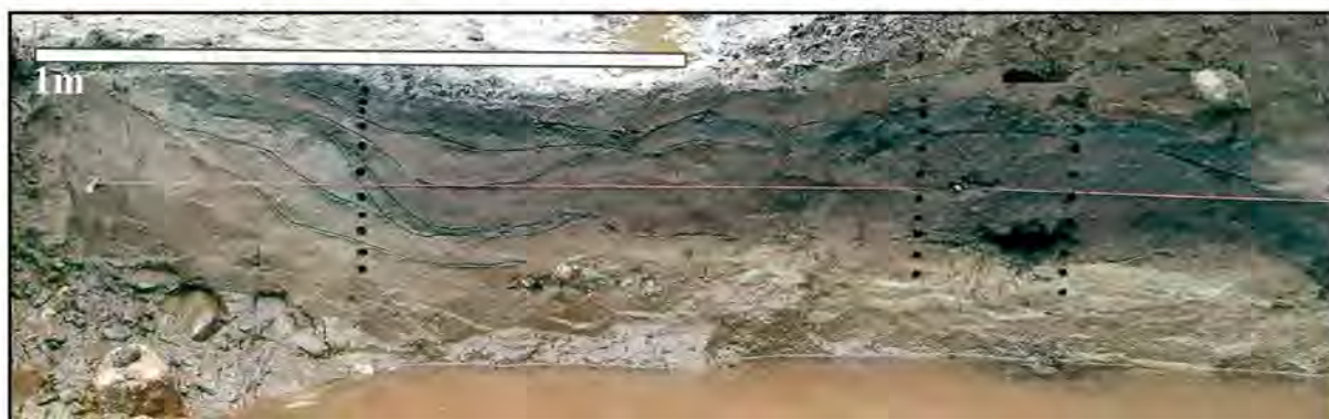
Fig. 26. Pollenprofil 1. Her vises tverrsnittet av bekkeleiet med den klare sedimenteringen i forsenkningen, samt uttaket av de ulike pollenseriene og ^{14}\text{C} -prøver.
