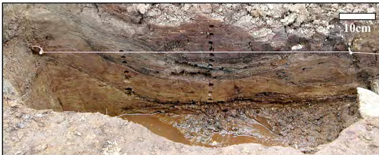
Fig. 27. Pollenprofil 2. Her vises tverrsnittet av bekkeleiet med den klare sedimenteringen i forsenkningen, samt uttaket av de ulike pollenseriene og ^{14}\text{C} -prøver.
