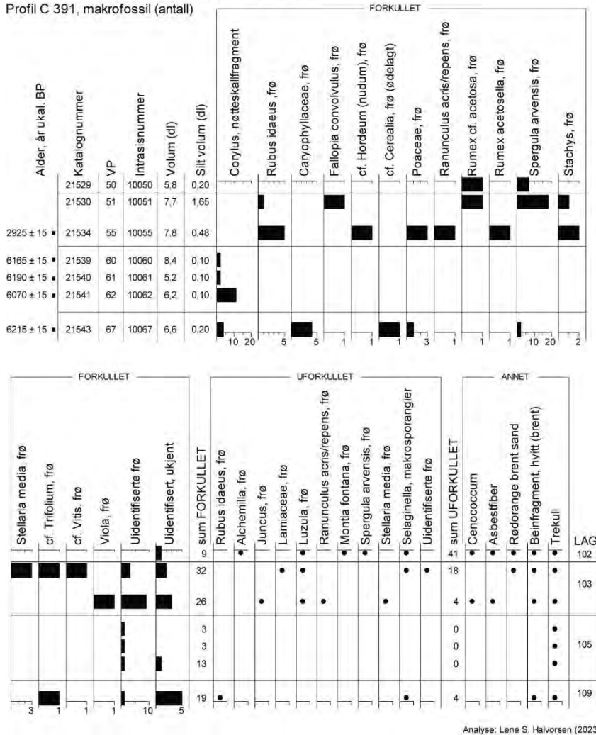
Figur 5. Profil C 391, makrofossilidiagram. Sorte stolper viser antall, prikker viser forekomst. Merk ulik faktor på x-aksen.
