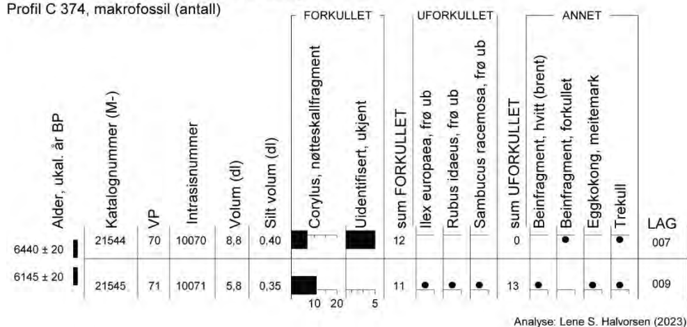
Figur 8. Profil C 374, makrofossildiagram.
