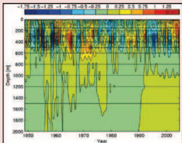
Figur 1. Temperatur (venstre) og saltanomalier (høyre) målt ved Stasjon M.
