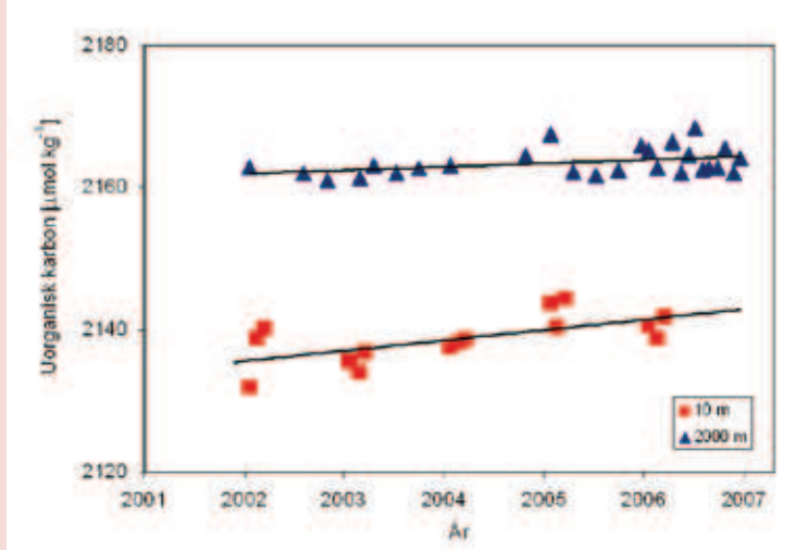
Figur 3. Viser hvordan det uorganiske karboninnholdet i havoverflaten (røde firkanter) og på 2000 m dyp (blå trekkanter) har økt over år. Overflatedata er fra vintermånedene januar, februar og mars. I dypet er organisk materiale brutt ned i sine enkelte bestanddeler (inkludert uorganisk karbon), og derfor er karbonverdiene der høyere enn i overflaten.
